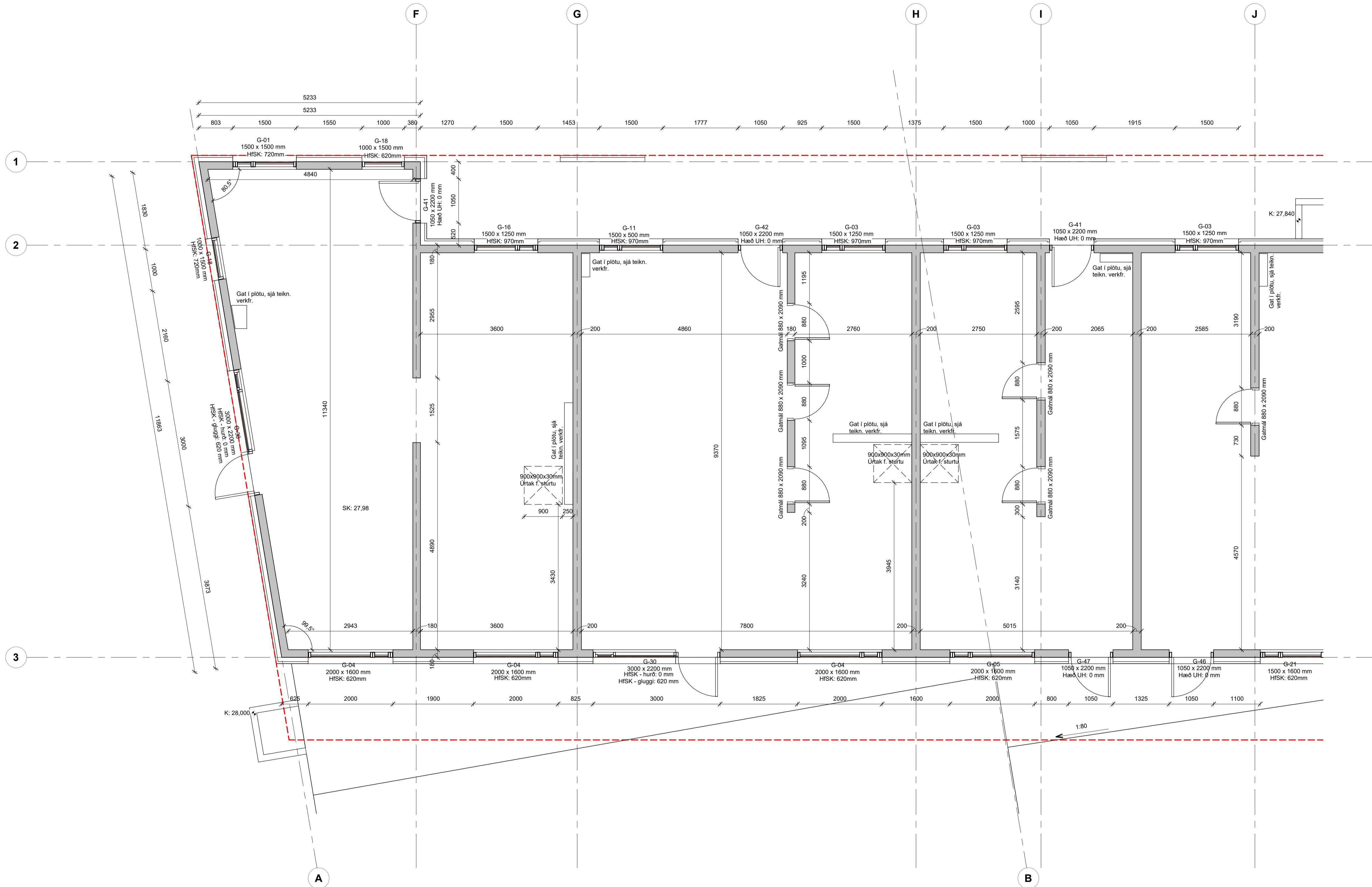
01-Hæð 1 - Steyputeikningar - Mhl. 02 - hluti 1 1:50
