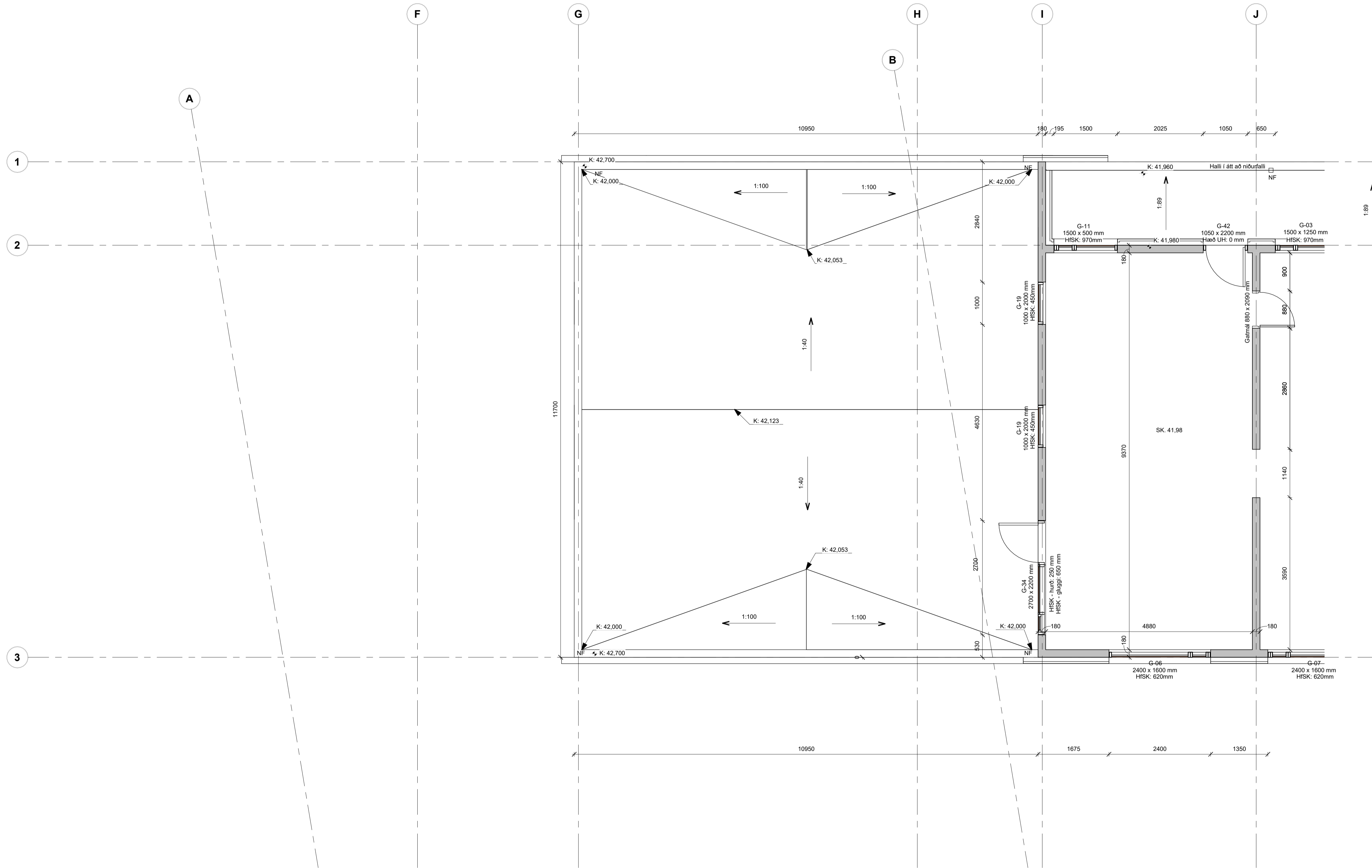
06-Hæð 6 - Steyputeikningar - Mhl. 02 - hluti 1 1 : 50
