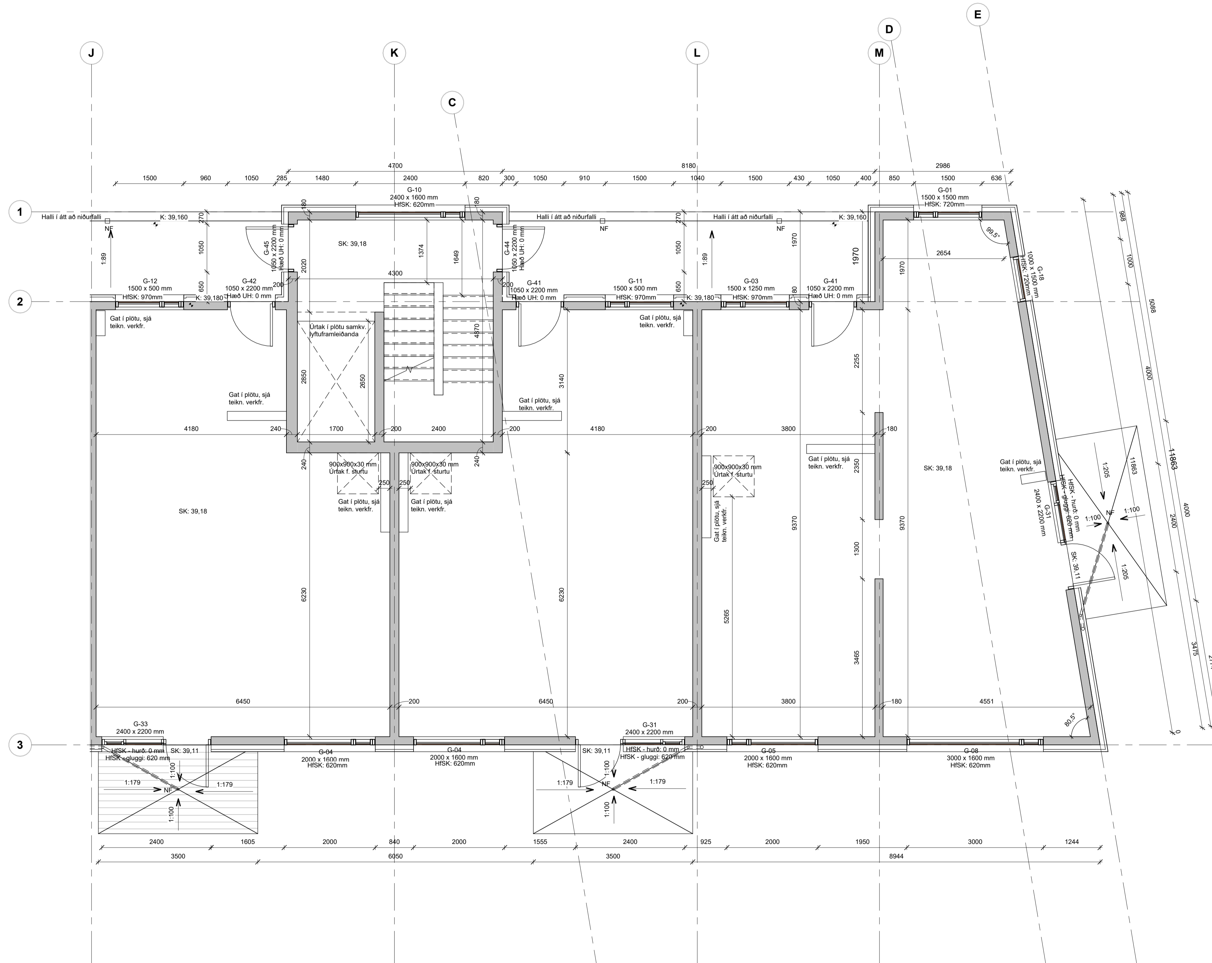
05-Hæð 5 - Steyputeikningar - Mhl. 02 - hluti 2 1 : 50
