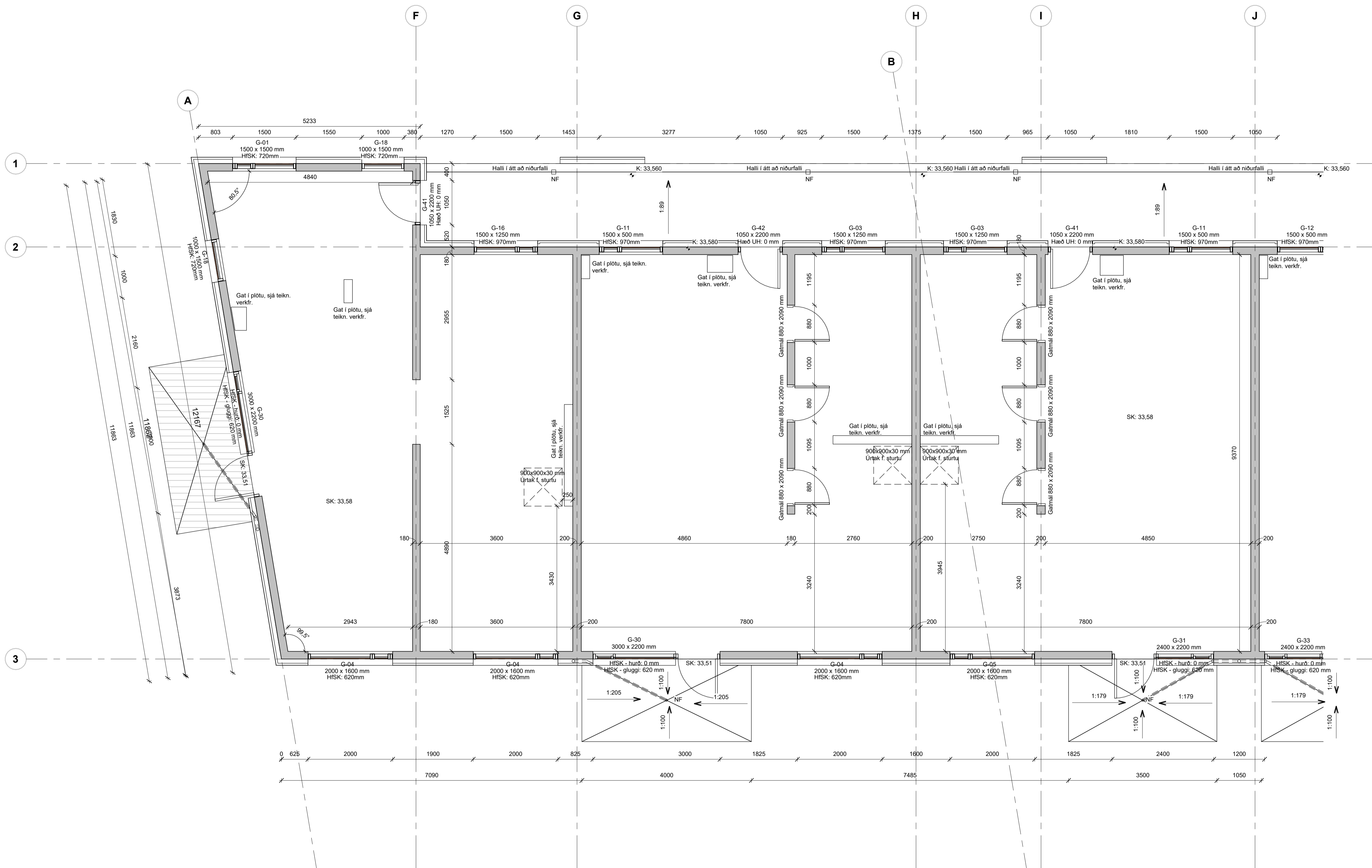
03-Hæð 3 - Steyputeikningar - Mhl. 02 - hluti 1
