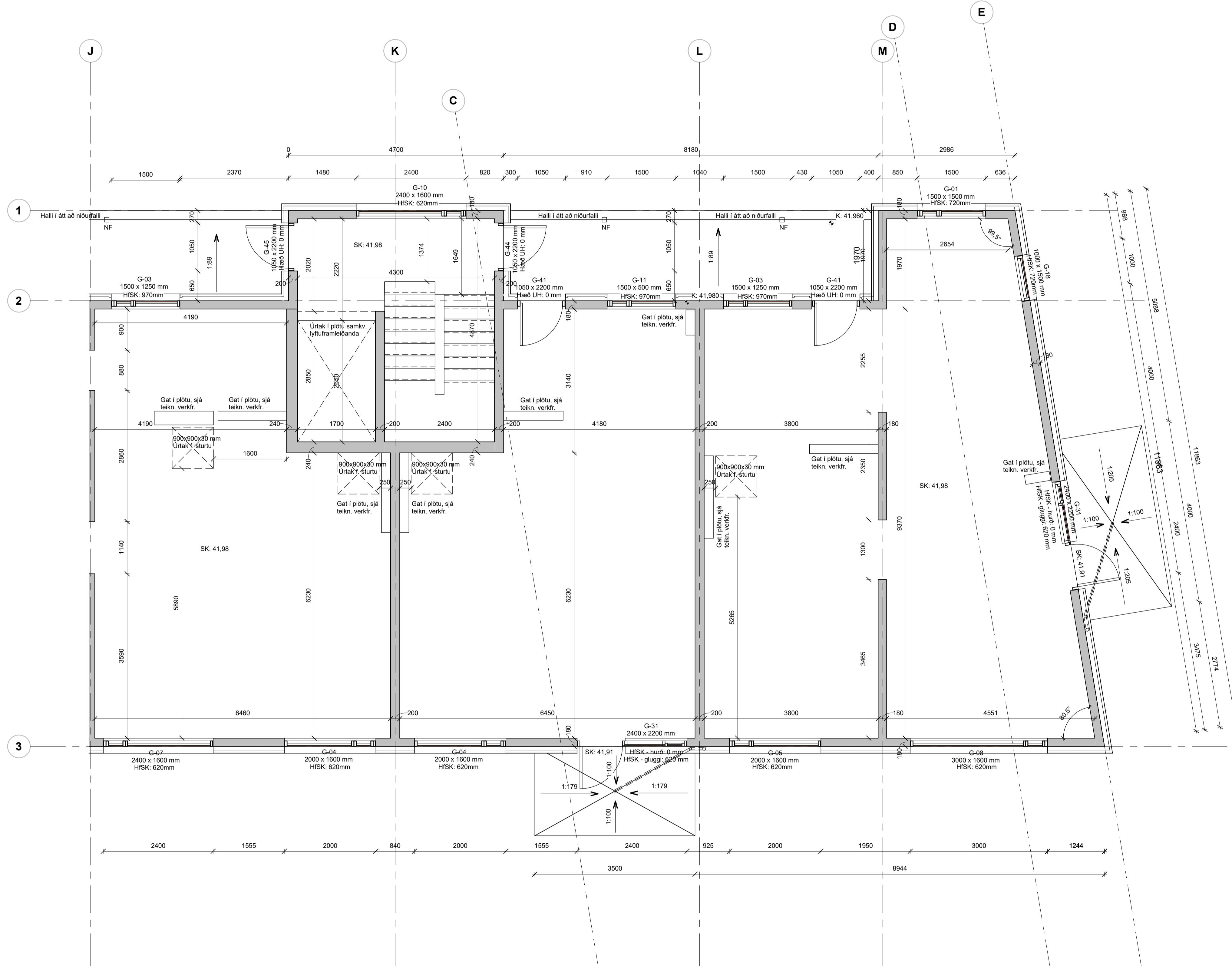
06-Hæð 6 - Steyputeikningar - Mhl. 02 - hluti 2 1 : 50
